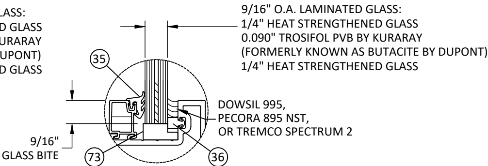
GLAZING DETAIL D1
