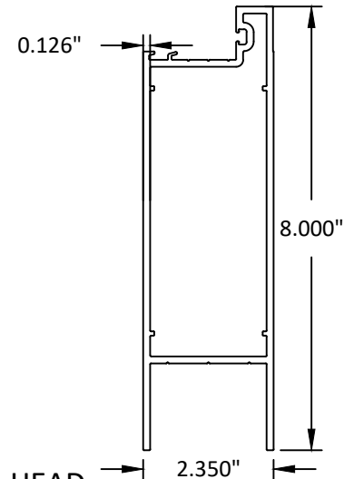
61 8" BOTTOM RAIL MONO. 6063-T5
