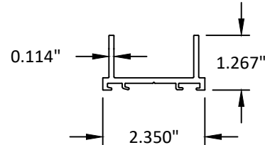
59 MIDRAIL FILLER 6063-T5
