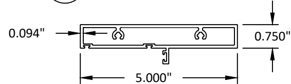
65 CW SUBFRAME - HEAD 6063-T5
