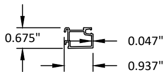
57 EXT. GLASS STOP-MONO. 6063-T5
